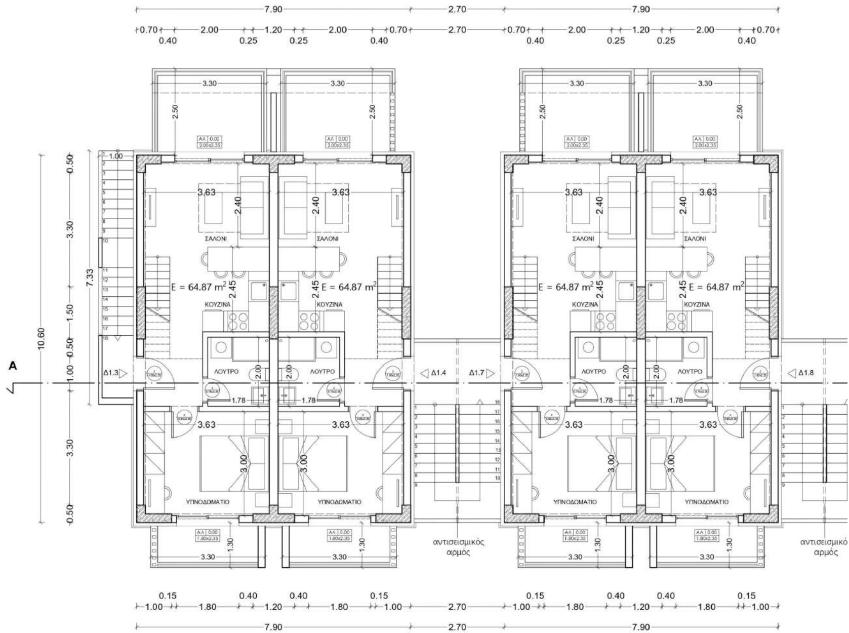
Κάτοψη Ορόφου κτιρίων 1Α, 1Β
