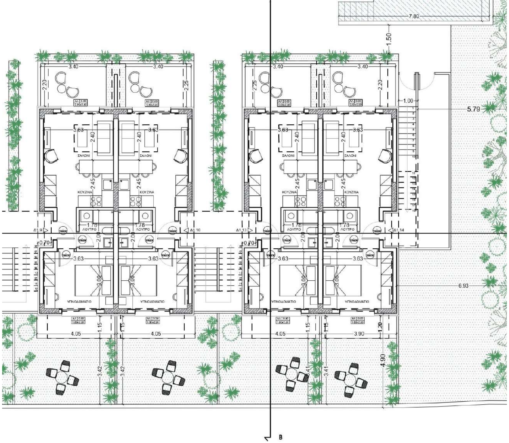
Κάτοψη Ισογείου κτιρίων 1Γ, 1Δ
