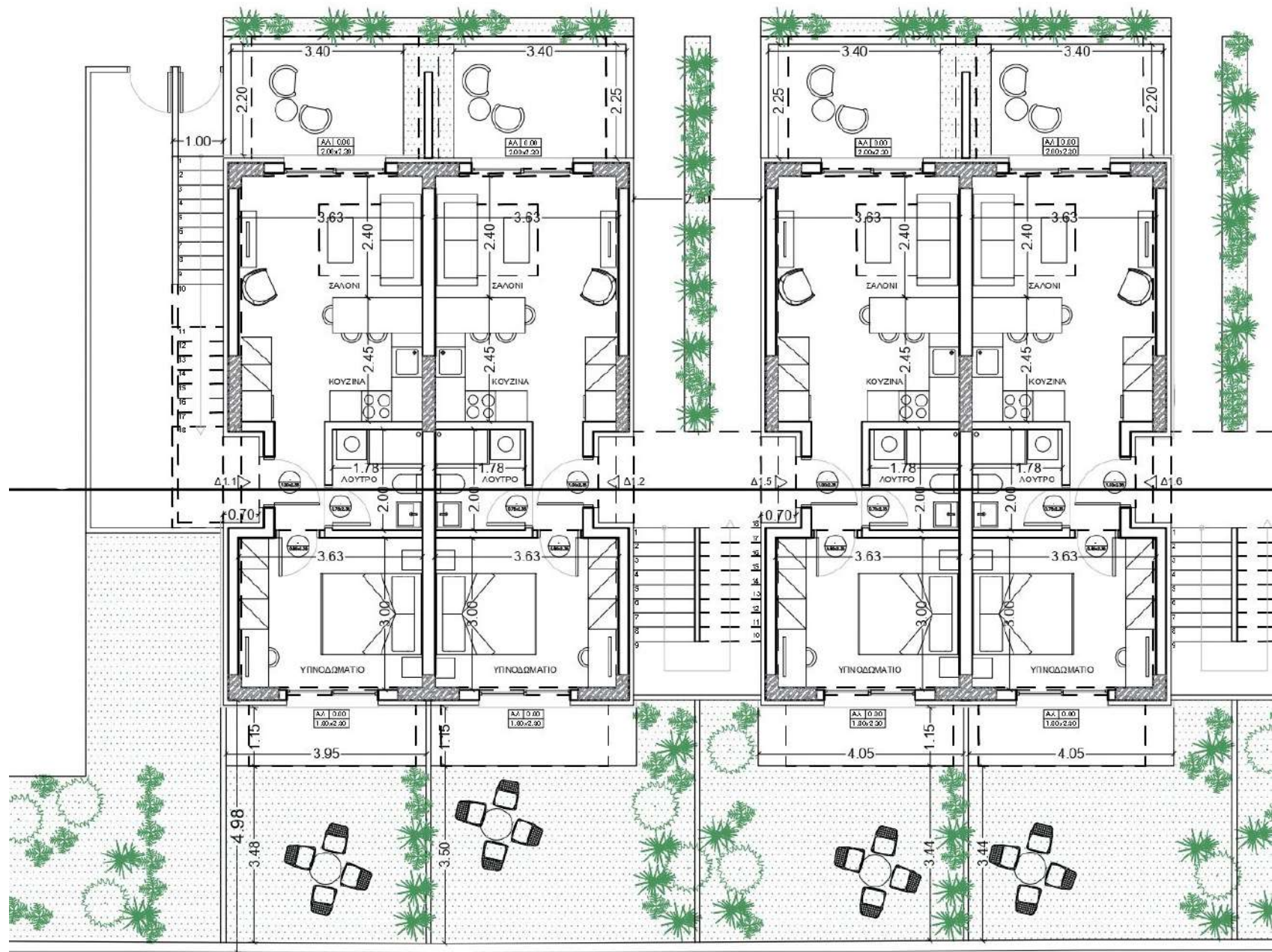
Κάτοψη Ισογείου κτιρίων 1Α, 1Β
