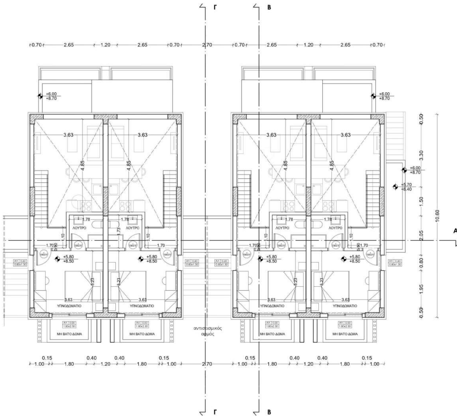
Κάτοψη Σοφίτας Κτιρίων 1Γ, 1Δ
