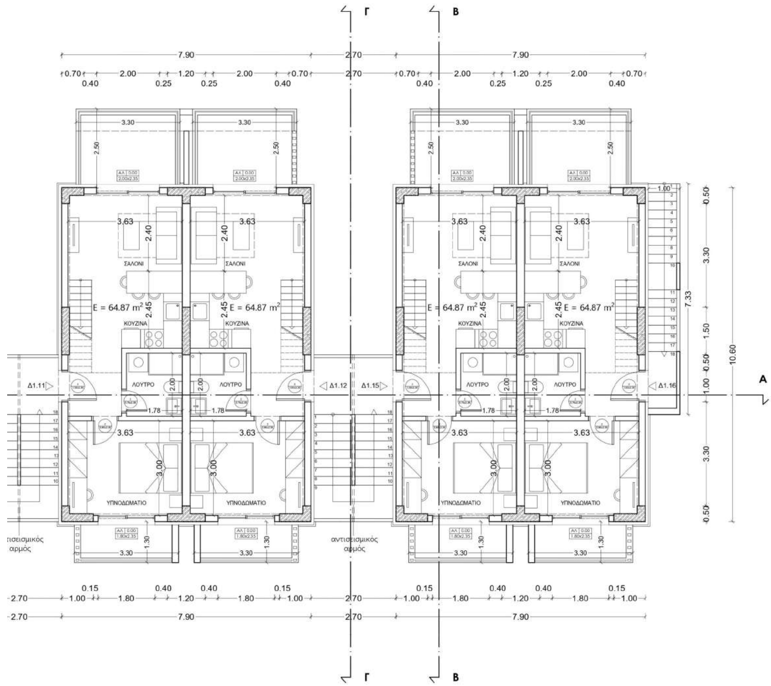
Κάτοψη Ορόφου κτιρίων 1Γ, 1Δ
